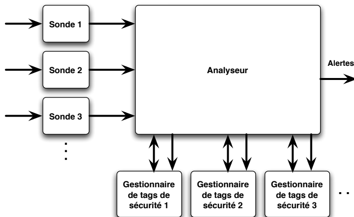
FIG. 3.2 – Architecture centralisée
