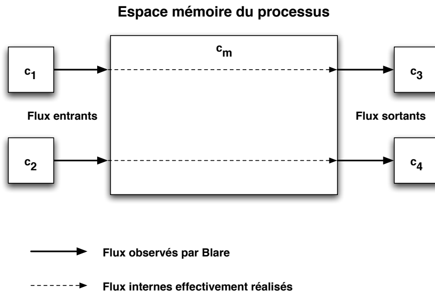
FIG. 3.7 – Flux d'informations internes effectivement réalisés
